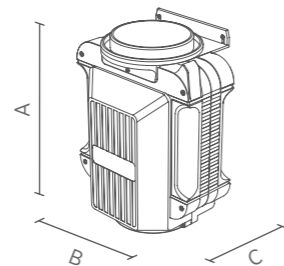
ASPIRODOR 165 Ø 100 - 120 mm
