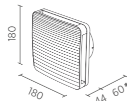
ONDA 12/5" Ø 120 mm
